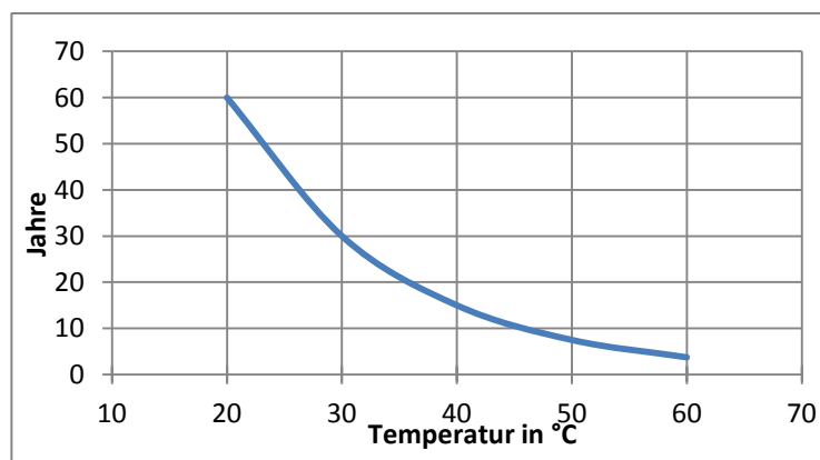
Abbildung 2: Lebensdauer in Abhängigkeit der Temperatur
